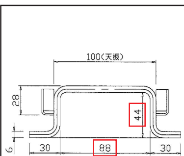
配線またぎ寸法 (mm) (88×44)
