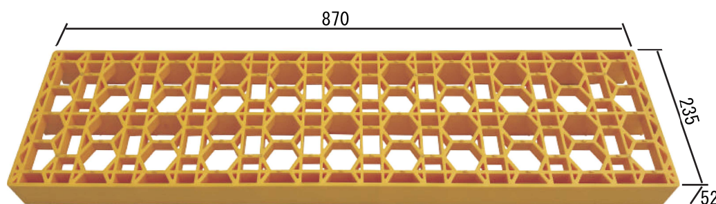
詳細寸法図
