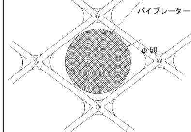
パイプレーターが通る形状
