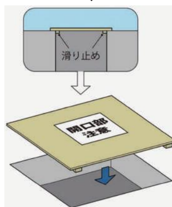
墜落防止措置 (開口部等)
