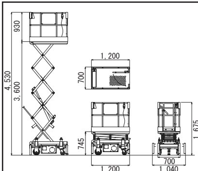
【LS36 詳細図】
