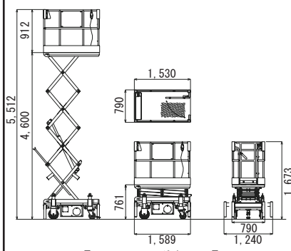
【VEGA46 詳細図】
