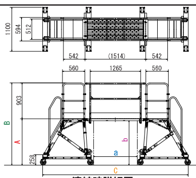
連結時詳細図
