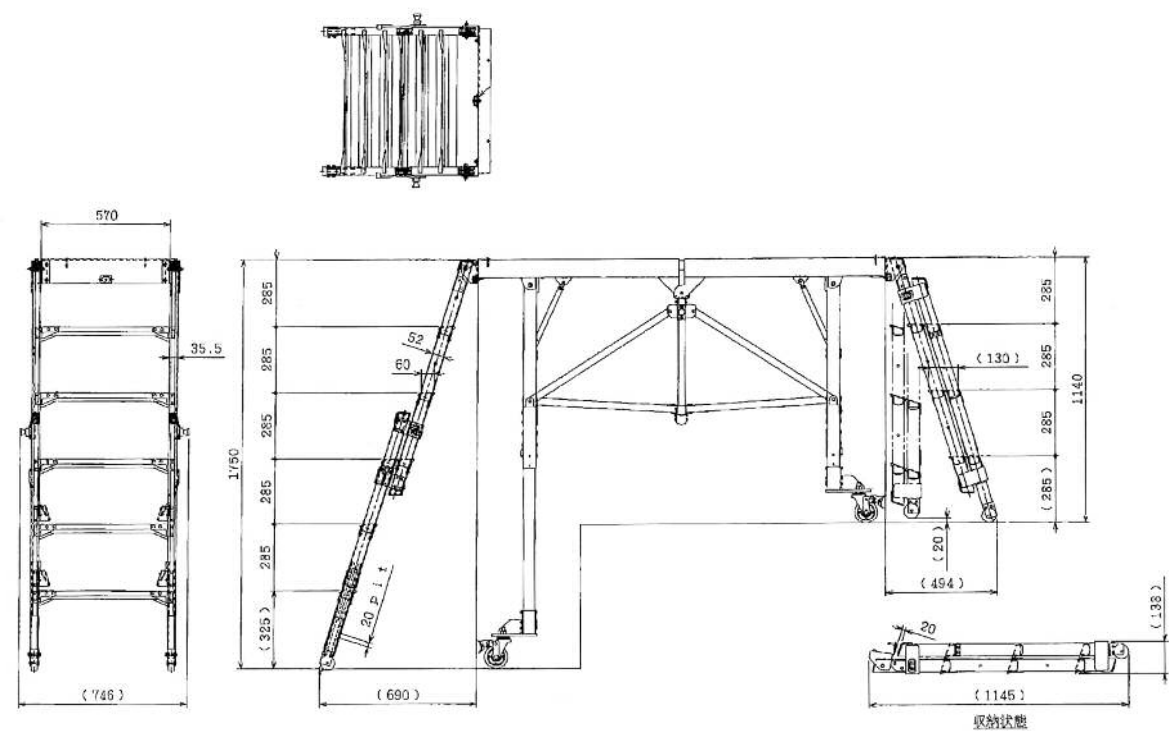
コンステージはしご(1750用)
