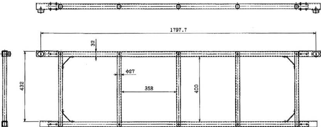
コンステージ連結手摺(1100・1750・1980用)
