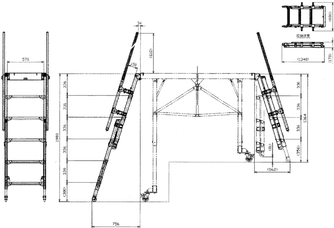
コンステージはしご(1980用)
