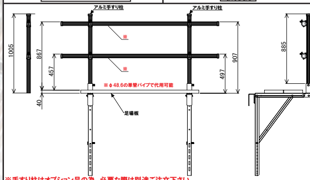
手すり柱 (アルミ製)
