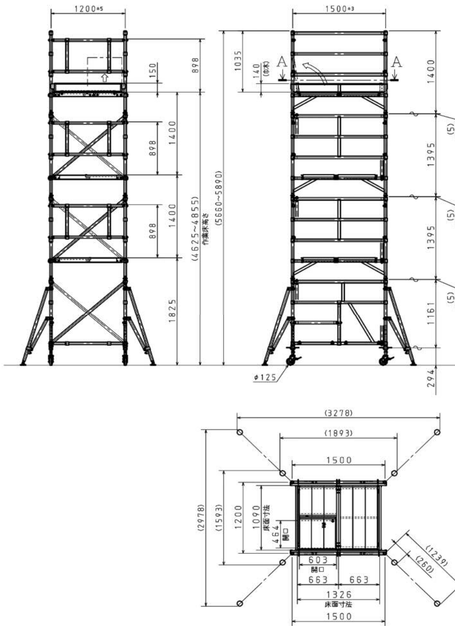
A-A矢視 アウトリガー寸法
