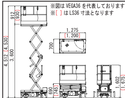
【LS36・VEGA36 詳細図】
