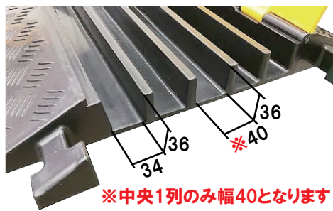
②PW-3PRO (φ34・36ケーブルまで対応)
