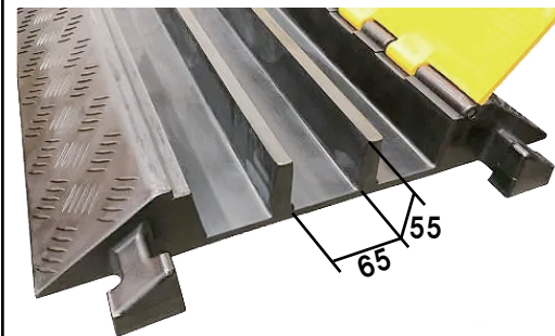
①PG-3PRO (φ55ケーブルまで対応)
