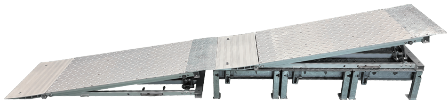
(例 2) アルミスロープ+アクトスロープ専用架台+アルミスロープ
