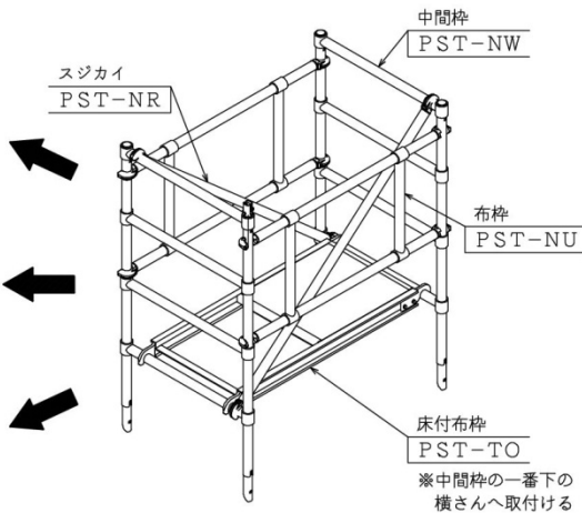
中階の組立
