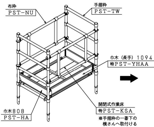
上階+巾木の組立
