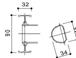
支柱・踏ざん詳細
